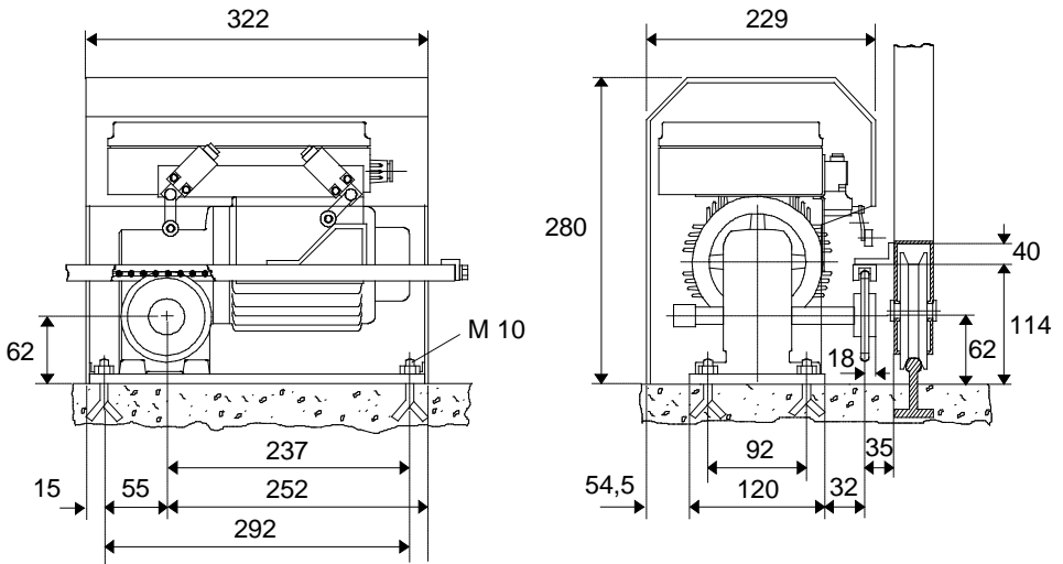
Bild 6 Maßbild der Typen WS 300/1, DS 400/1 und DS 600/1 mit Kettenschiene und Kettenrad
