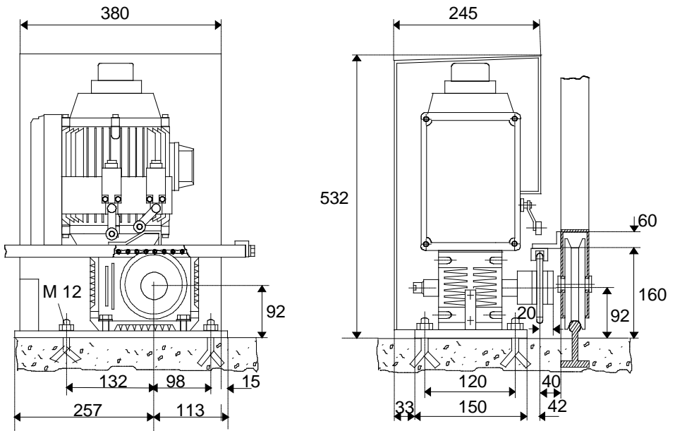
Bild 6 Maßbild der Typen WS 300/1, DS 400/1 und DS 600/1 mit Kettenschiene und Kettenrad
